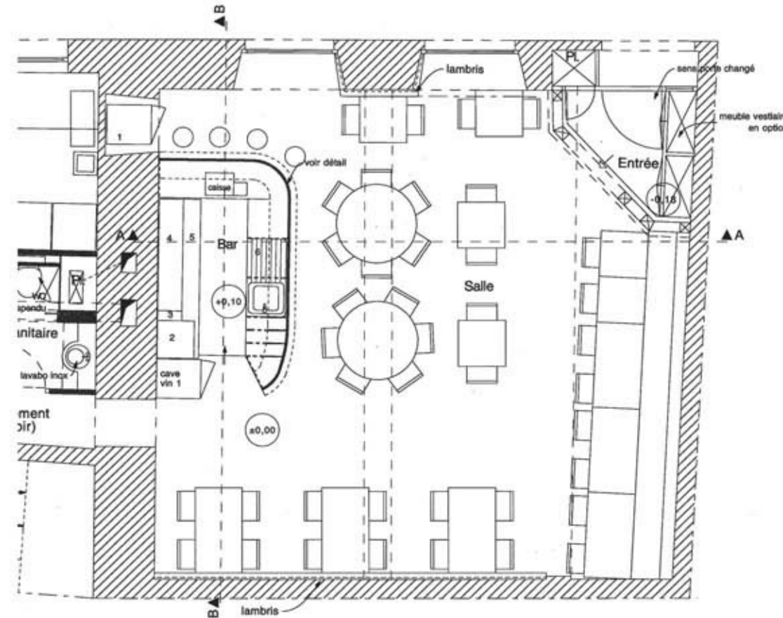
Plan d'aménagement
